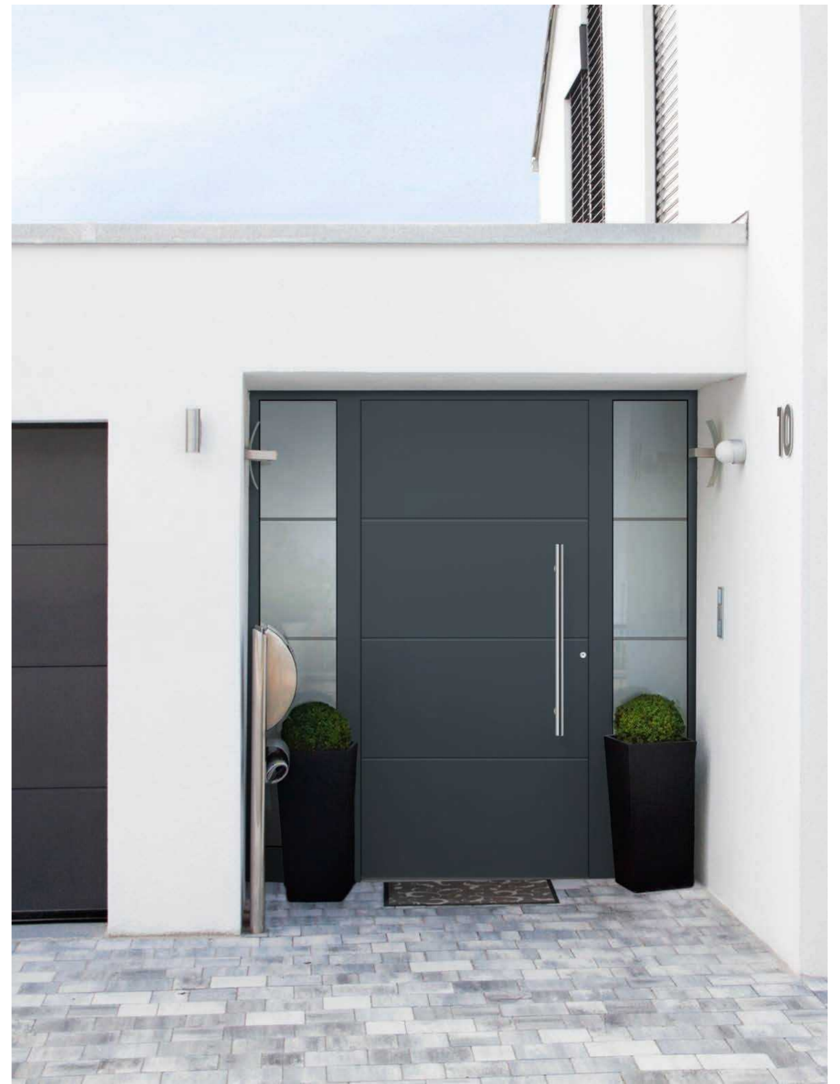
Modell E-243 FD T: KÖtherm 96 mit Seitenteilen, 0683-7016 Feinstruktur F: Nutenfräsung nur außen G: Motivverglasung 1443 Z: Handhabe 23150
