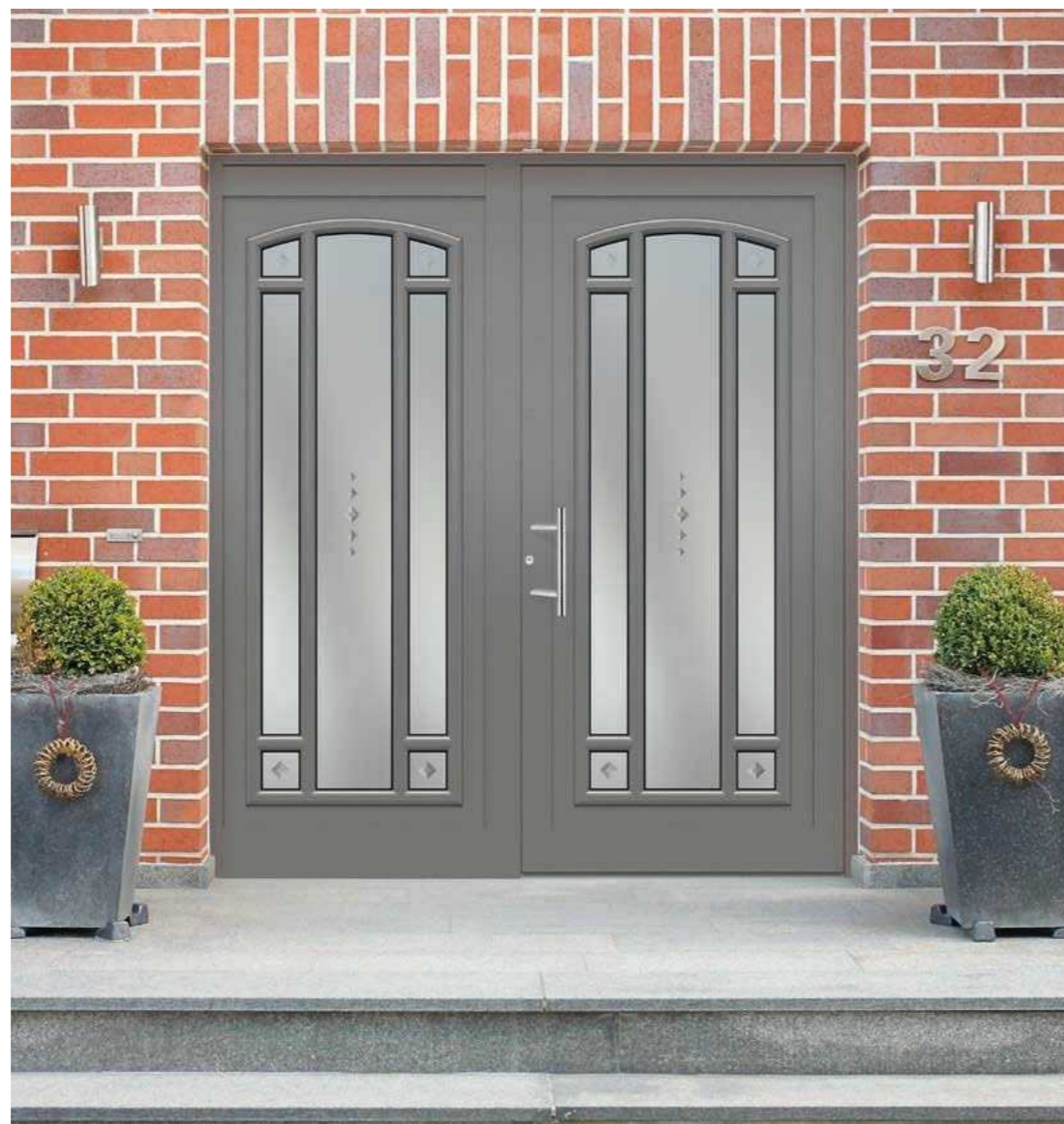
van Gogh 61 PL T: K0therm 96 mit Seitenteil, RAL 9007 F: eingesetzt G: Motivverglasung 1200 Z: Handhabe 22109
